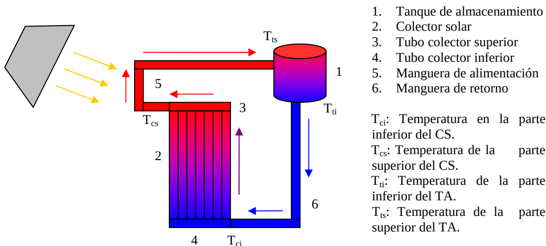
Figura 1: Esquema del sistema de calentamiento solar de agua, su funcionamiento con indicación de color para las temperaturas (roja, mayor, azul, menor), y ubicación de los puntos de medición.
