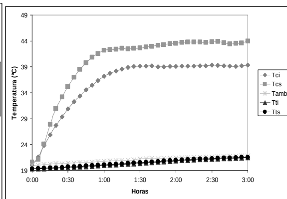
Figura 17: Medición de temperaturas con una radiación incidente de 600 \text{ W/m}^2 y aislamiento térmico
