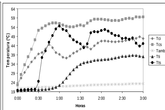
Figura 19: Medición de temperaturas con una radiación incidente de 850 \text{ W/m}^2 y aislamiento térmico
