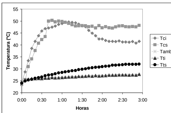
Figura 11: Medición de temperaturas con una radiación incidente de 750 W/m 2
