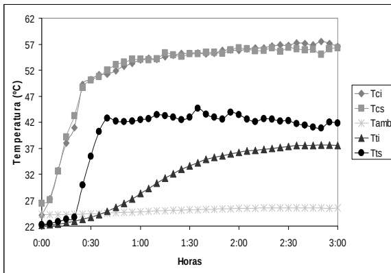
Figura 16: Medición de temperaturas con una radiación incidente de 1000 \text{ W/m}^2
