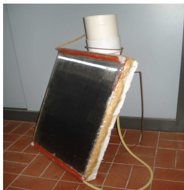
Figura 3: Fotografía del equipo empleado.
