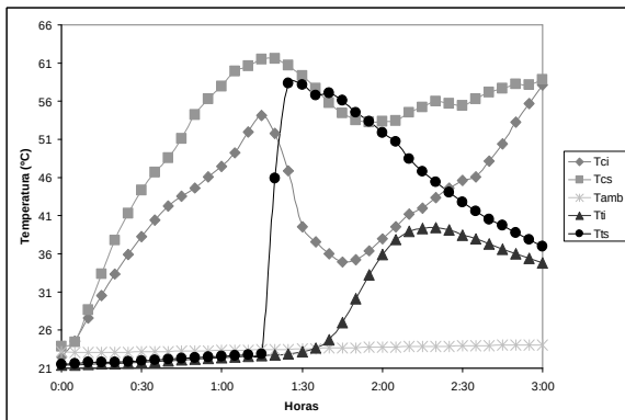
Figura 18: Medición de temperaturas con una radiación incidente de 800 \text{ W/m}^2 y aislamiento térmico
